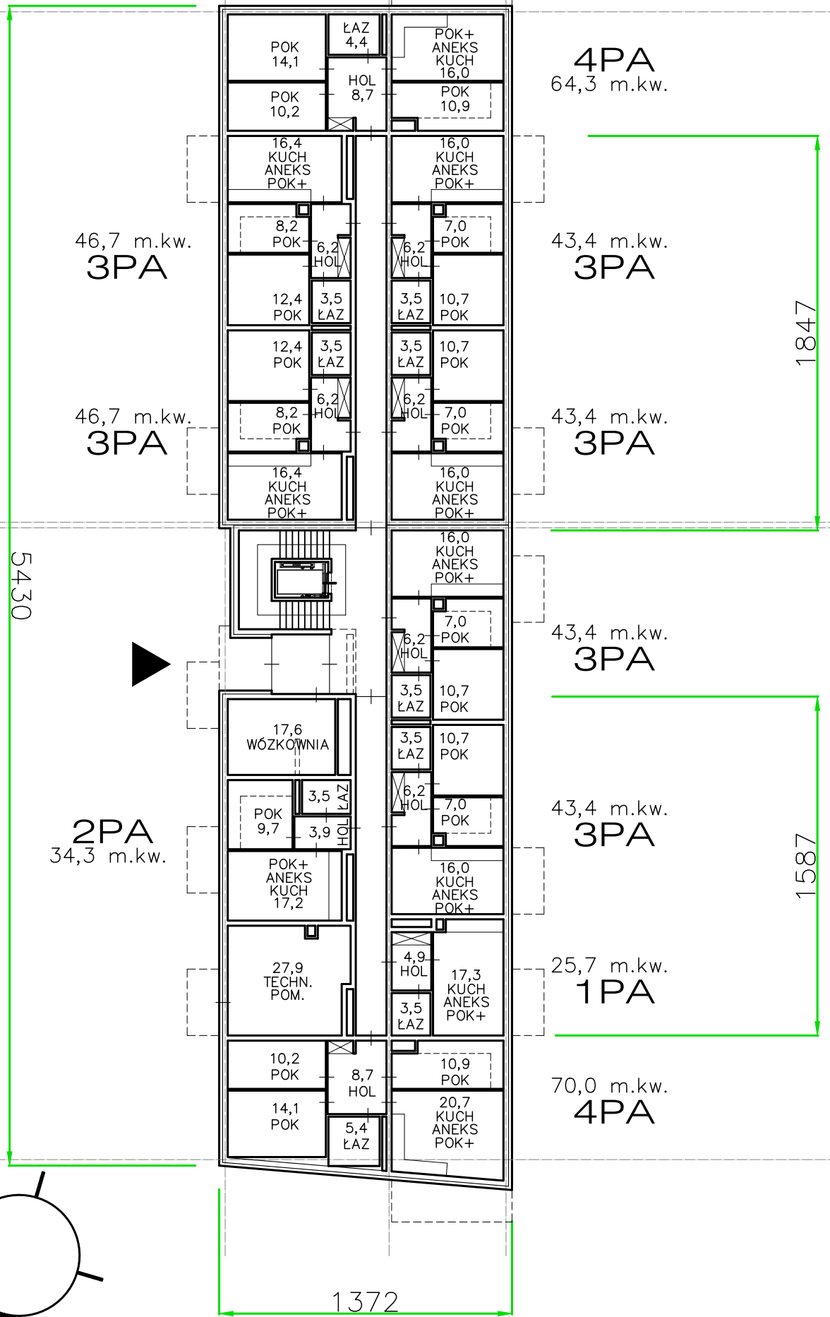
KONDYGNACJA 1
