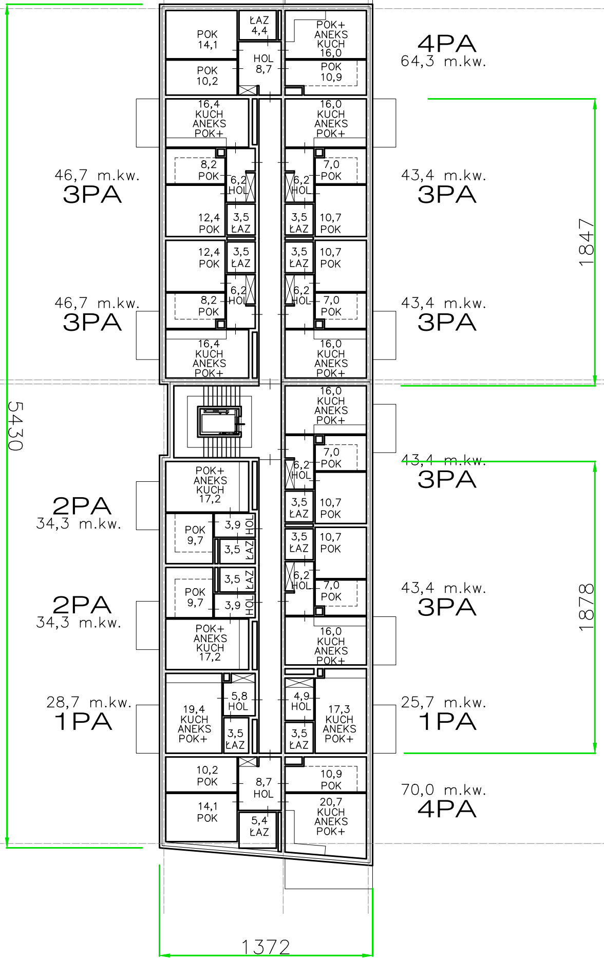
KONDYGNACJA 2, 3, 4
